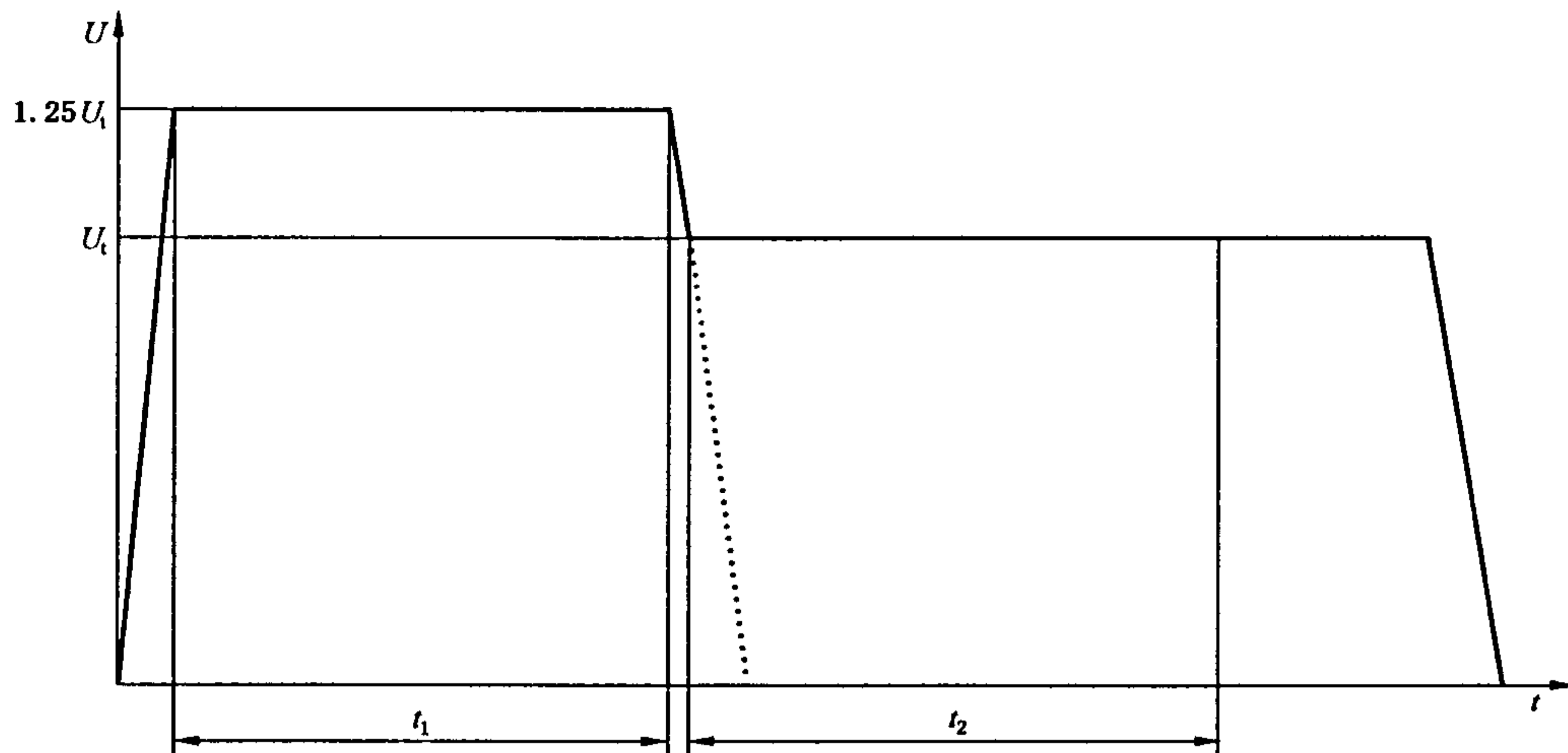
图3 试验电压
