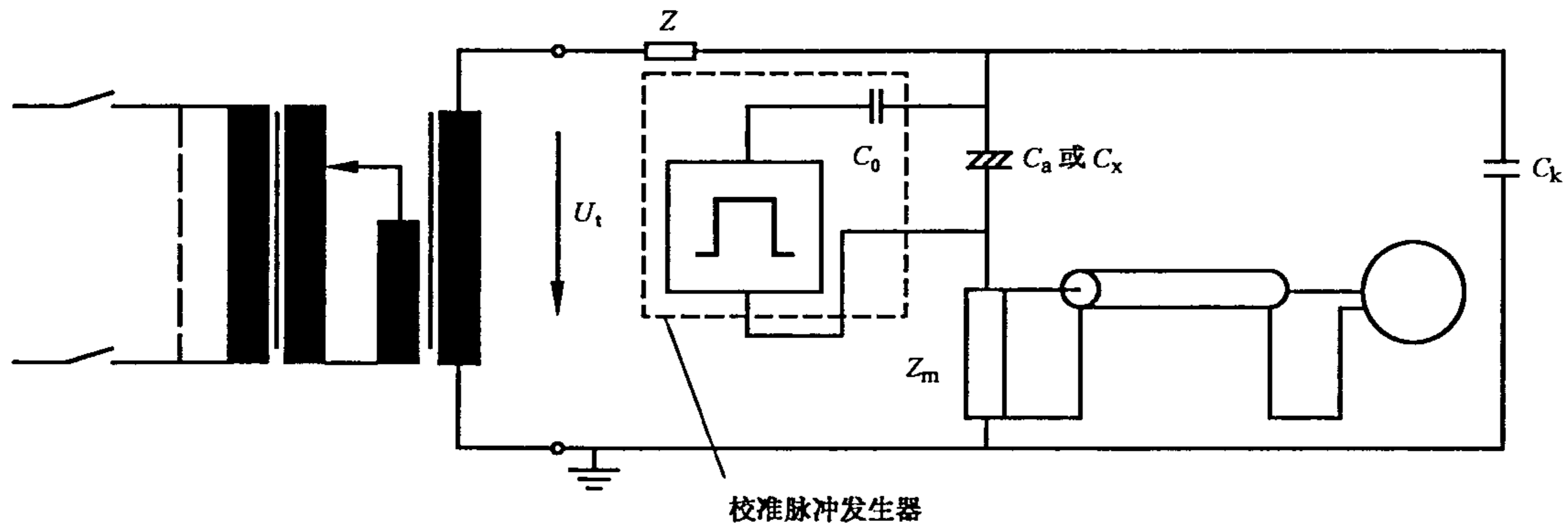
图 C.4 不接地试品的校准
