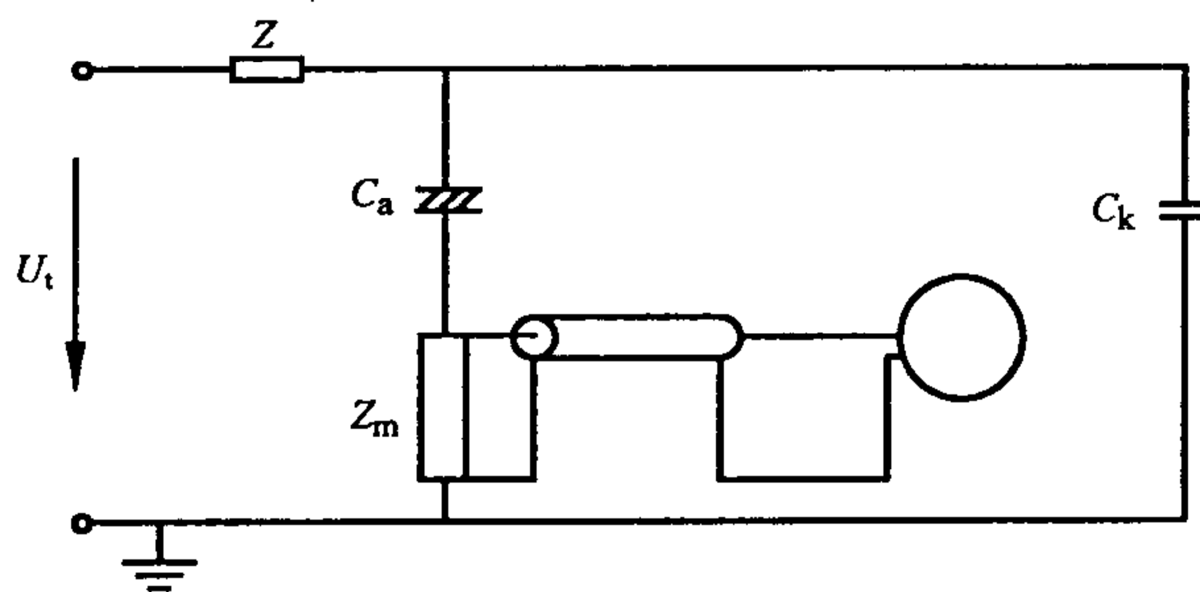
图 C.2 不接地试品
