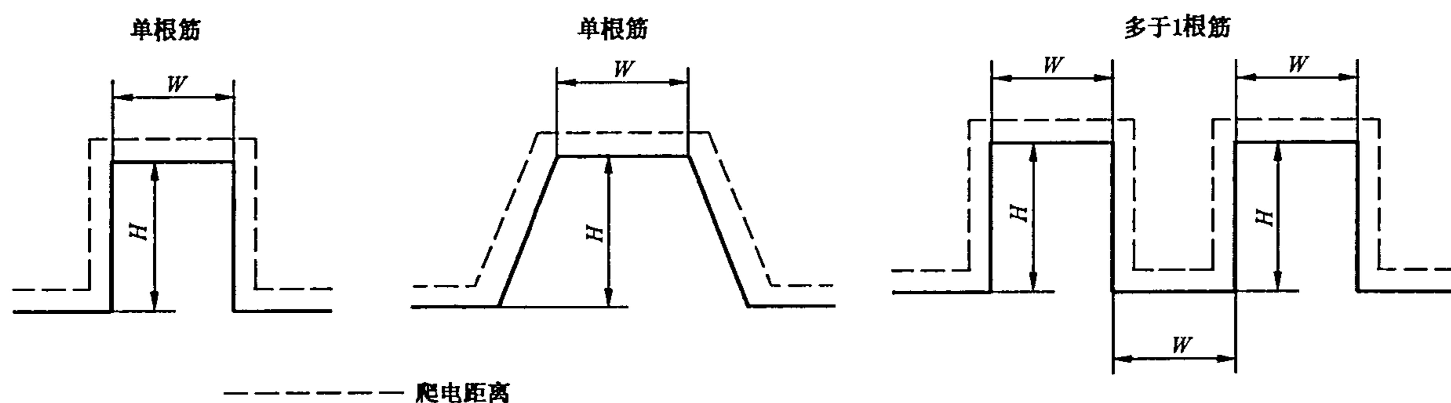
图 2 筋的宽度( W )和高度( H )尺寸
