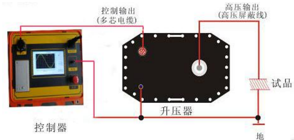
图 3 接线示意图
