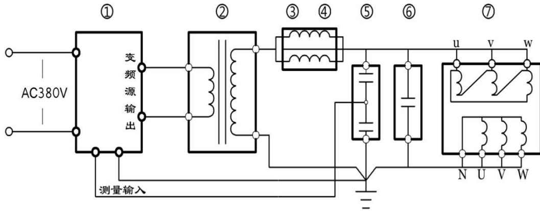
变压器耐压试验接线图
