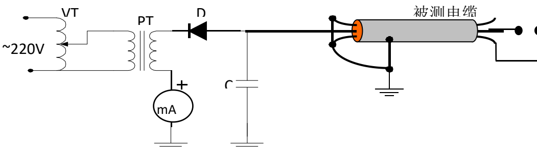
图 28 球间隙放在终端的接线图
