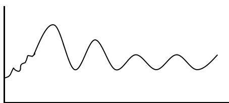
图 21 闪络测量法未扩展的波形
