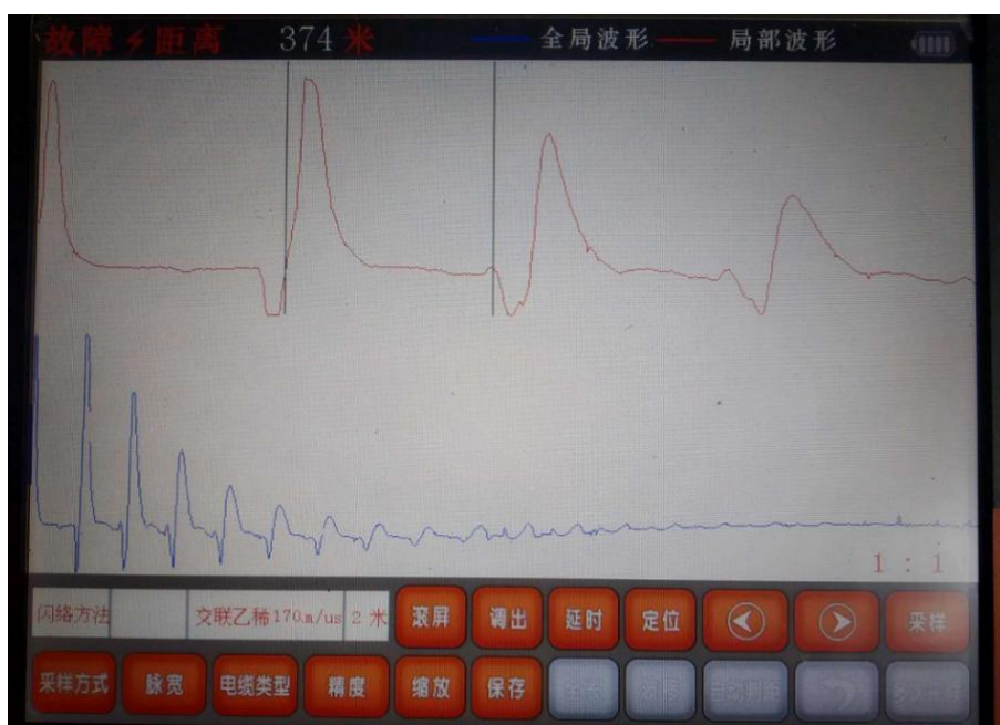
冲击闪络法测试波形示例
