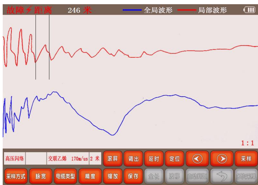
冲击闪络法测试波形示例
