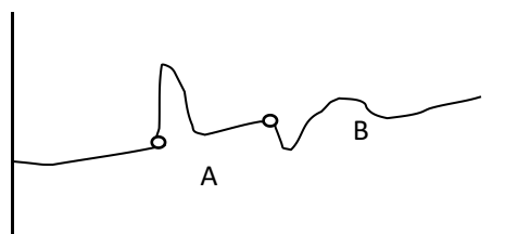
图 22 闪络测量法已扩展的波形
