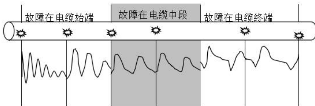
闪络法测试波形的变化规律图
