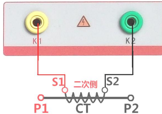
图 5，CT 励磁特性接线图
