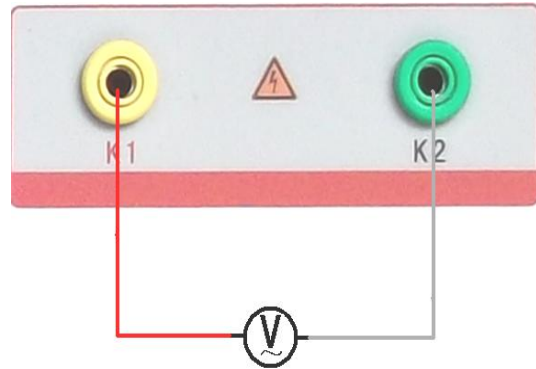
图 43，电压校准接线图
