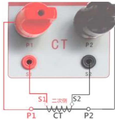
图 13, CT 变比极性 (角差比差) 接线图
