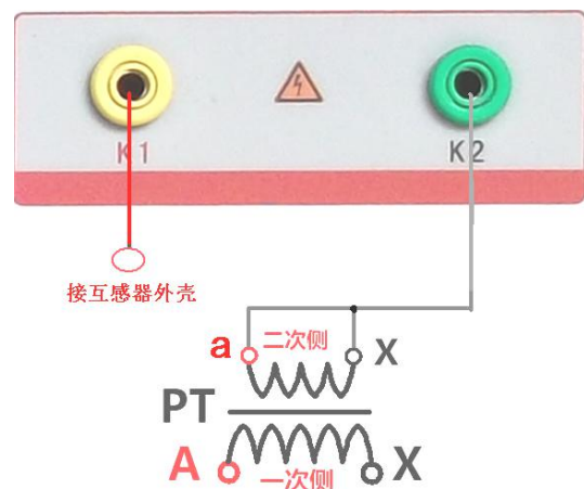
图 33， PT 交流耐压接线图
