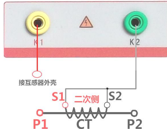
图 19, CT 交流耐压接线图
