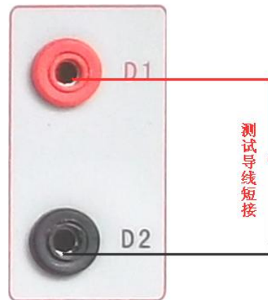
图 23，导线阻值清零接线图
