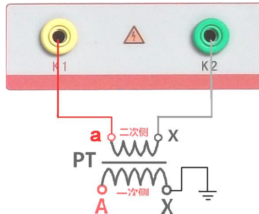
图 26，PT 励磁特性接线图
