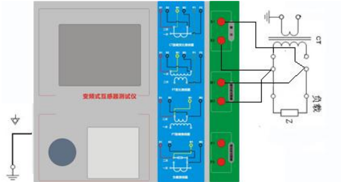
图 2.2 CT 二次负荷试验接线方式
