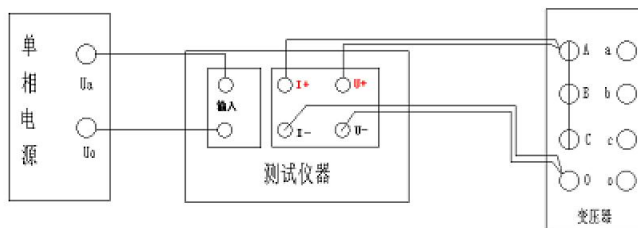
零序阻抗直接接线图
