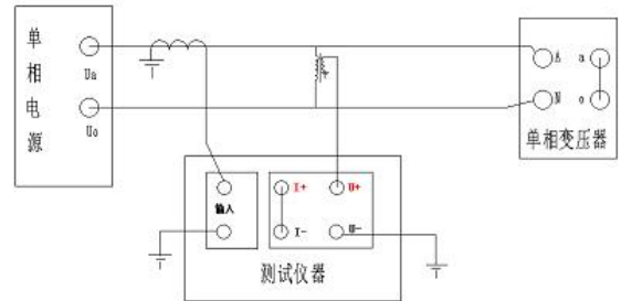
外接电压、电流互感器接线图
