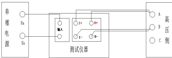
单相变压器直接接线图
