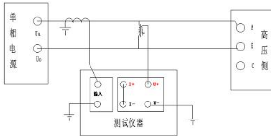
星接-单相外接电压互感器和电流互感器接线图
