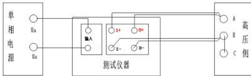
\Delta 接-直接接线图
