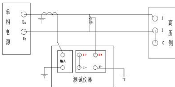
\Delta 接-外接电压互感器、外接电流互感器接线图
