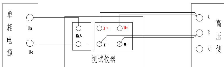
星接-单相直接接线图
