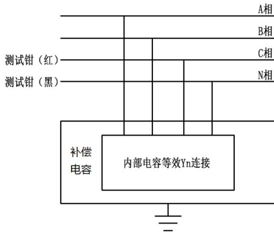
C 相接线
