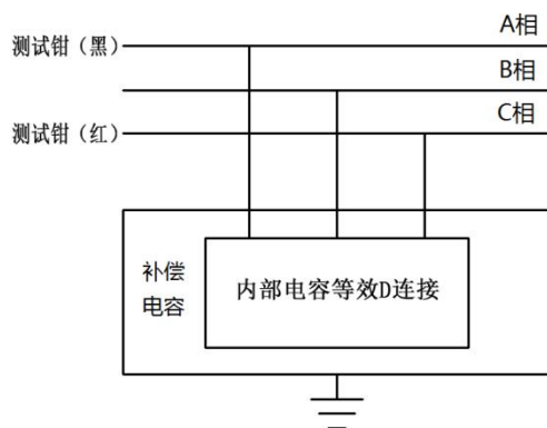
A相接线
