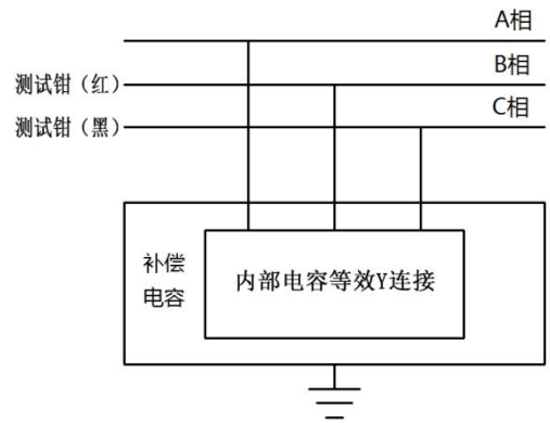
B 相接线
