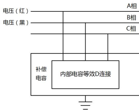
A相接线
