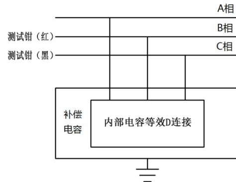
B相接线
