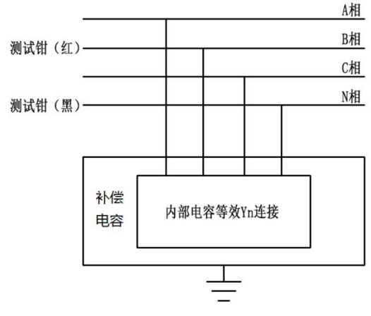
B相接线
