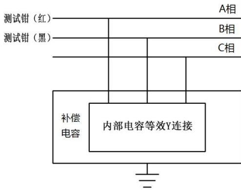
A 相接线
