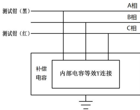
C 相接线
