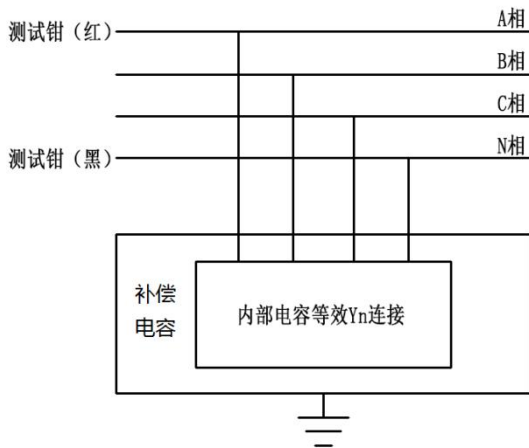
A相接线
