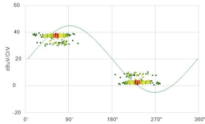
PRPD 图谱
