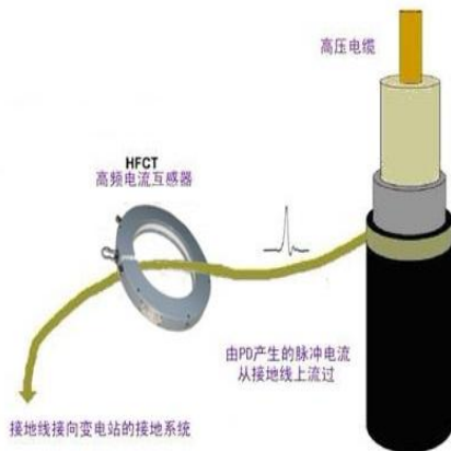
HFCT 接线方式
