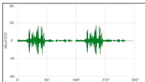
时域信号波形
