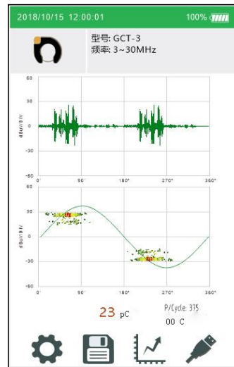
HFCT 测试界面
