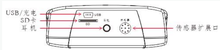
传感器扩展口
