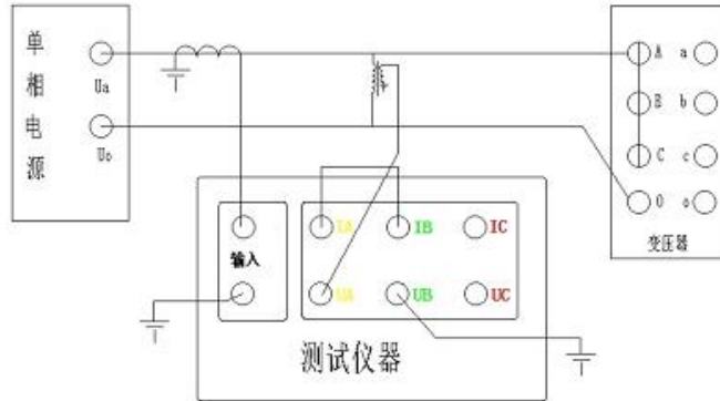
零序阻抗外接电压互感器、外接电流互感器接线图
