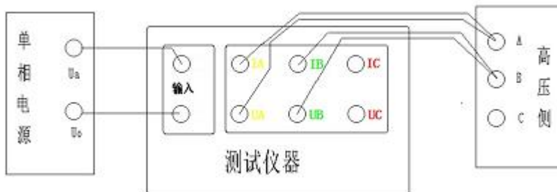
星接-单相直接接线图
